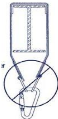
圖 9 打結轉接器的小 D 形環應穿過大 D 形環 應僅將連接子系統連接到小 D 形環。 請勿將該子系統同時連接到這兩個 D 形環。
